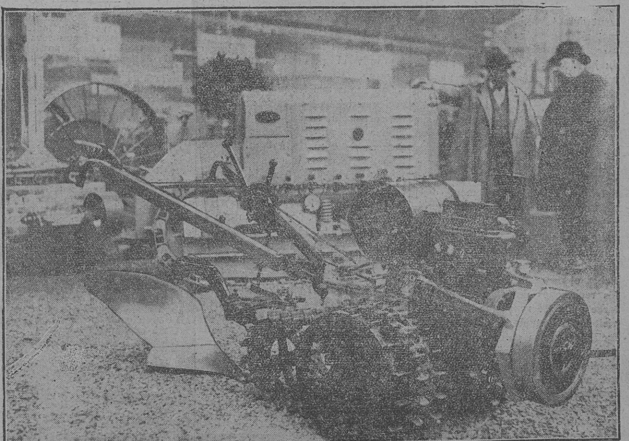
Charrue autochenille-mue par un moteur de 8 chevaux (un seul homme peut la conduire).
